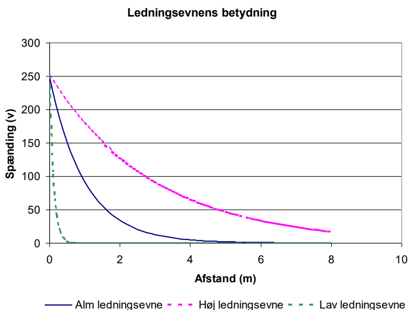
Figur 2. Spændingsfaldet i forhold til elektrodeafstanden i vand med forskellig ledningsevne.
