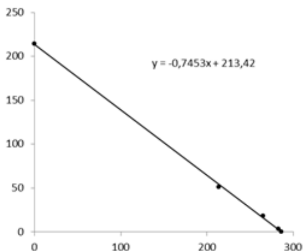
Figur 15. Grafisk metode til bestemmelse af bestandsstørrelse på basis af mindst to befiskninger. Punkterne for hver befiskning afsættes med en y-værdi, svarende til den enkelte fangst i befiskningen, mens x-værdien er summen af de tidligere fangster.
